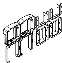
Supports intermédiaires
