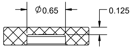
SECTION A-A SCALE 1 : 1
