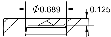
SECTION A-A SCALE 1 : 1
